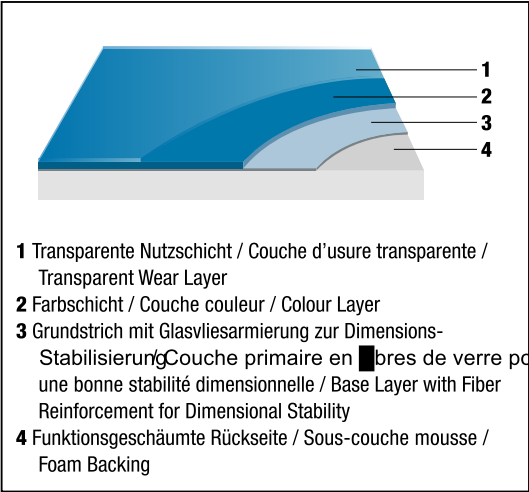
Bodenaufbau / Construction du tapis / Layer Structure
